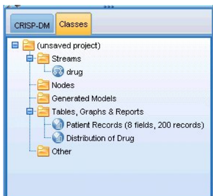
图 9. “类”视图
